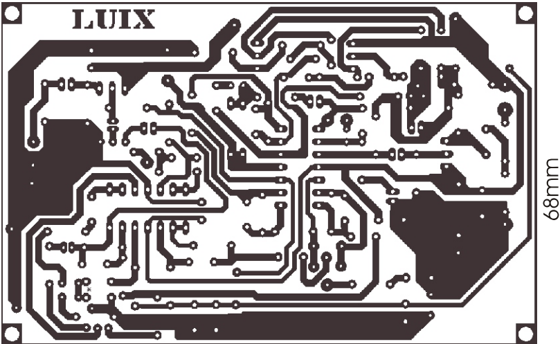
Pcb Invertida 107mm
